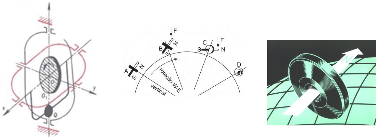
figura 3.27. Giroscópio forçado
