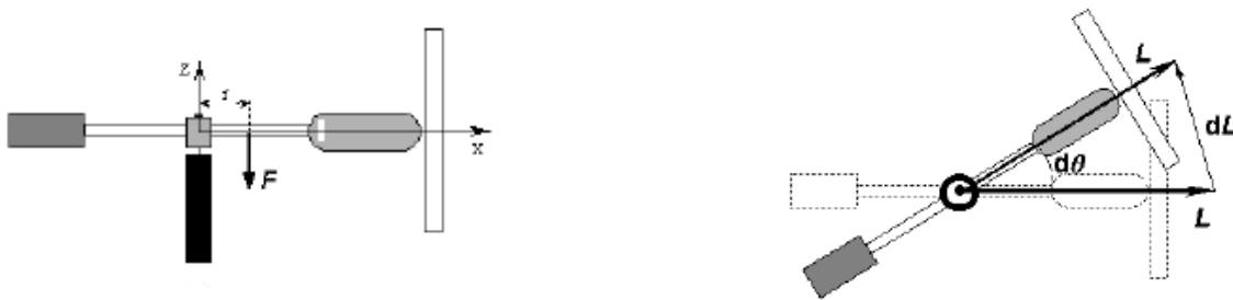
figura 3.24. Giroscópio forçado
