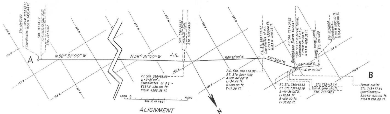
figura 3.51. Exemplo: representação em planta do túnel Eucumbene-Tumut, Austrália
